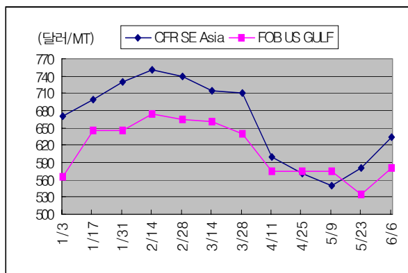
2-EH 가격추이(2003)
