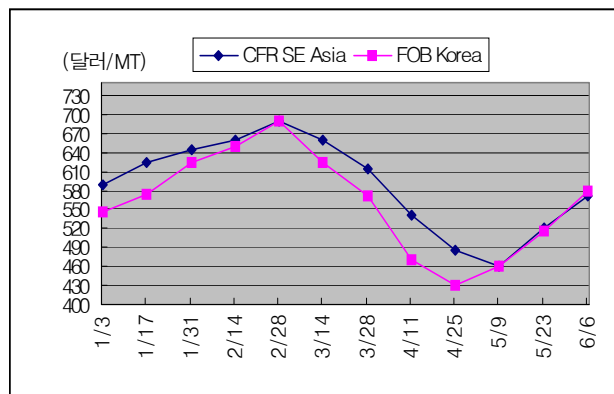
Propylene 가격추이(2003)
