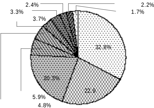
< 2> CO2 (1860~1990)
