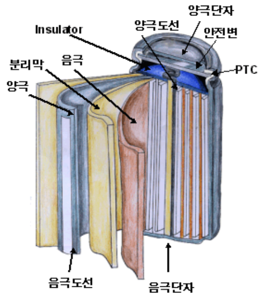
리튬이온전지 단면도
